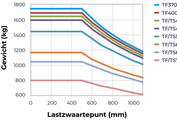
TF/TS-mast/enkel massief/vork van 900 mm/geen hulpstuk
