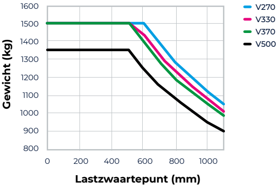
V-mast/enkel massief/vork van 900 mm/geen hulpstuk
