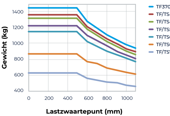
TF/TS-mast/enkel massief/vork van 900 mm/geïnt. zijverschuiver
