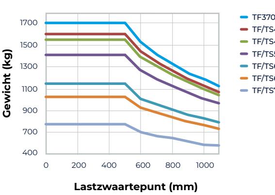
TF/TS-mast/enkel massief/vork van 900 mm/geïnt. zijverschuiver
