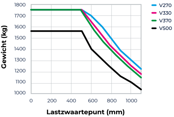
V-mast/enkel massief/vork van 900 mm/geïnt. zijverschuiver
