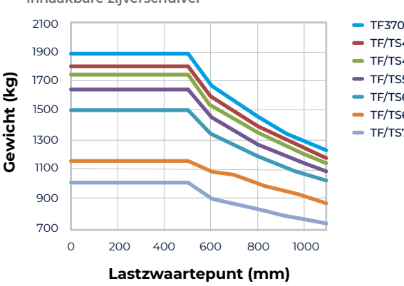
TF/TS-mast/enkel massief/vork van 900 mm/inhaakbare zijverschuiver
