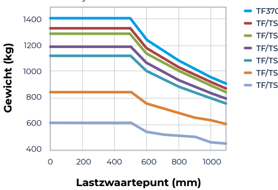
TF/TS-mast/enkel massief/vork van 900 mm/inhaakbare zijverschuiver
